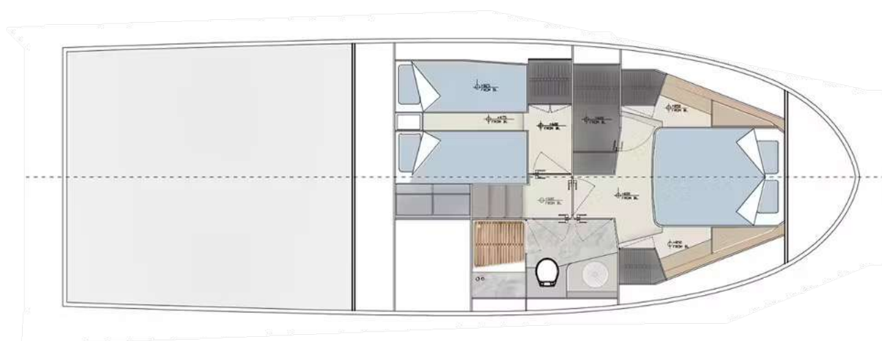
НИЖНЯЯ ПАЛУБА С
