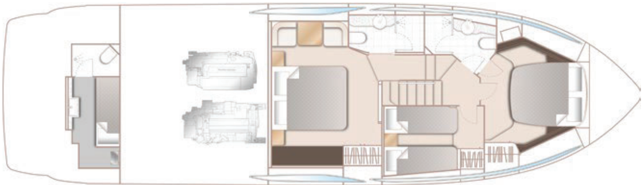
НИЖНЯЯ ПАЛУБА
