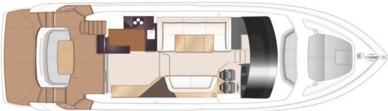
ГЛАВНАЯ ПАЛУБА
