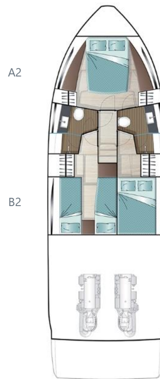
Нижняя палуба опциональная
