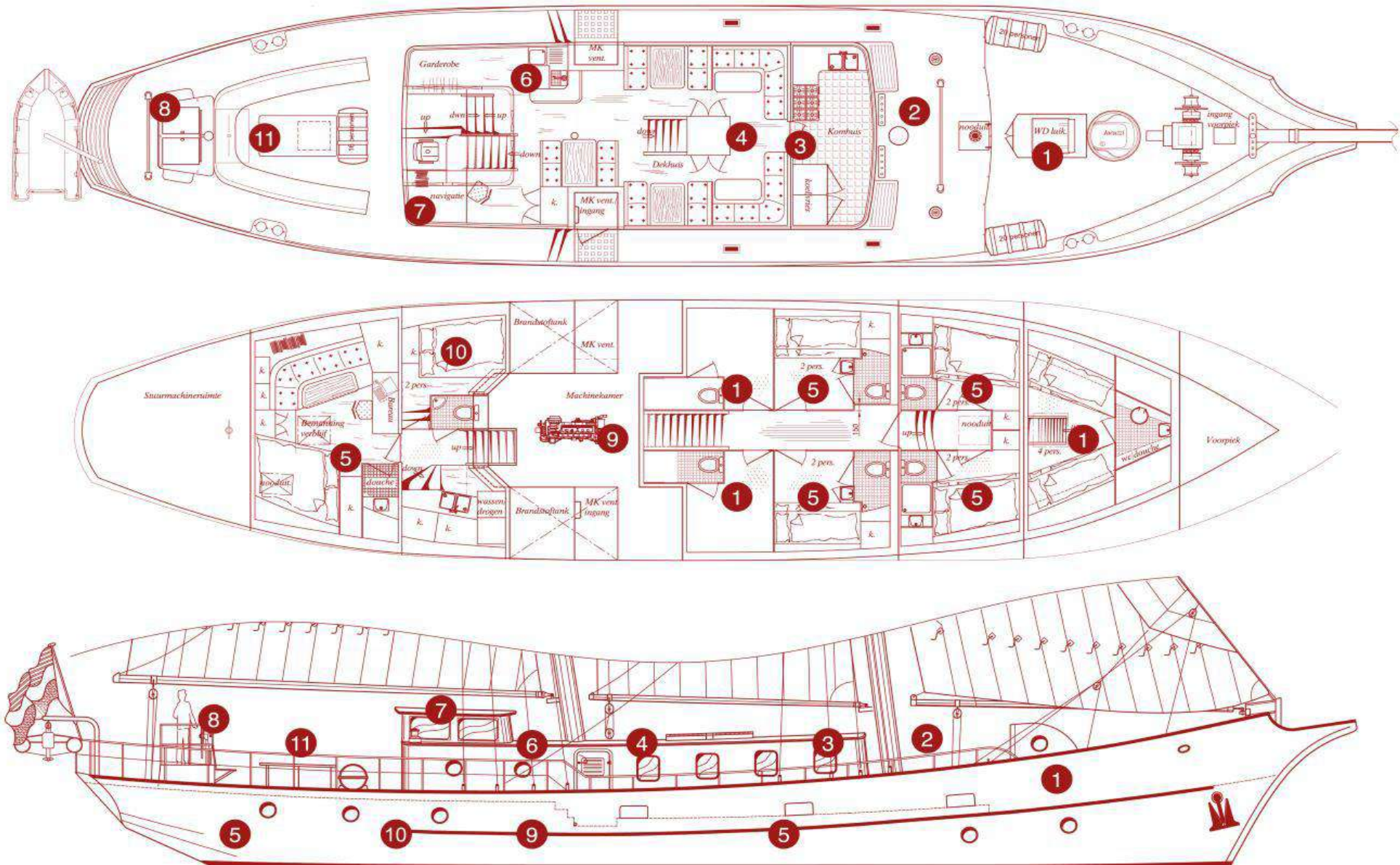
(1) Каюты экипажа; (2) Носовая зона отдыха; (3) Камбуз; (4) Ресторан; (5) Гостевые каюты; (6) Бар; (7) Рубка; (8) Флайбридж; (9) Машинное отделение; (10) Каюта капитана; (11) Кокпит
