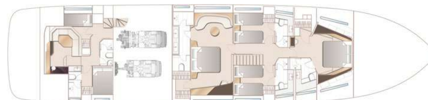
НИЖНЯЯ ПАЛУБА С ОПЦИОНАЛЬНОЙ КОРМОВОЙ ЗОНОЙ ОТДЫХА И КАЮТОЙ ЭКИПАЖА
