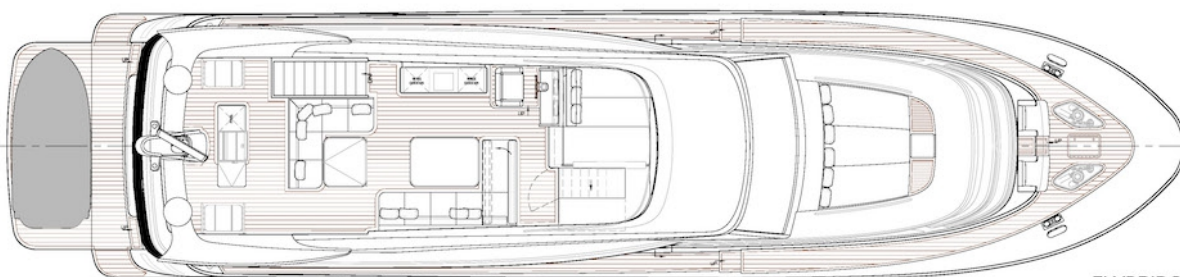
FLYBRIDGE
